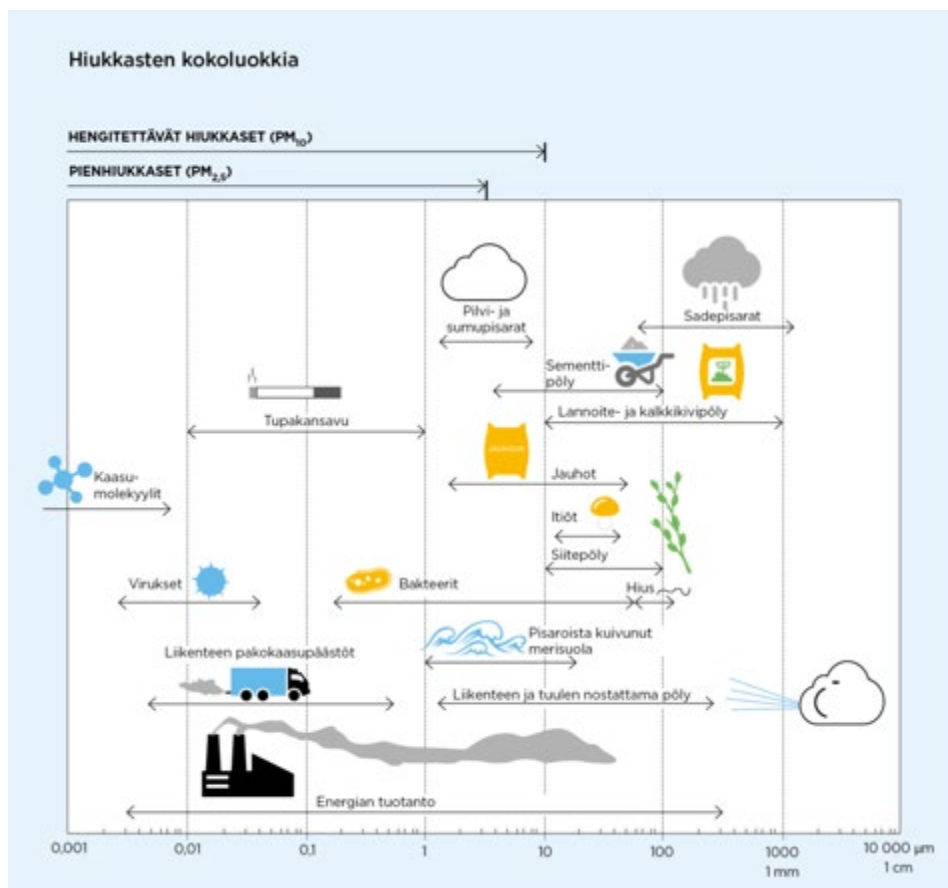
Kuva 37. Hiukkasten kokoluokkia. Hiukkasten koko ilmaistaan halkaisijana mikrometreissä ( \mu\text{m} ). Mikro ( \mu ) etuliite tarkoittaa miljoonasosaa. 1 \mu\text{m} on siten metrin miljoonasosa eli millimetrin tuhannesosa.
