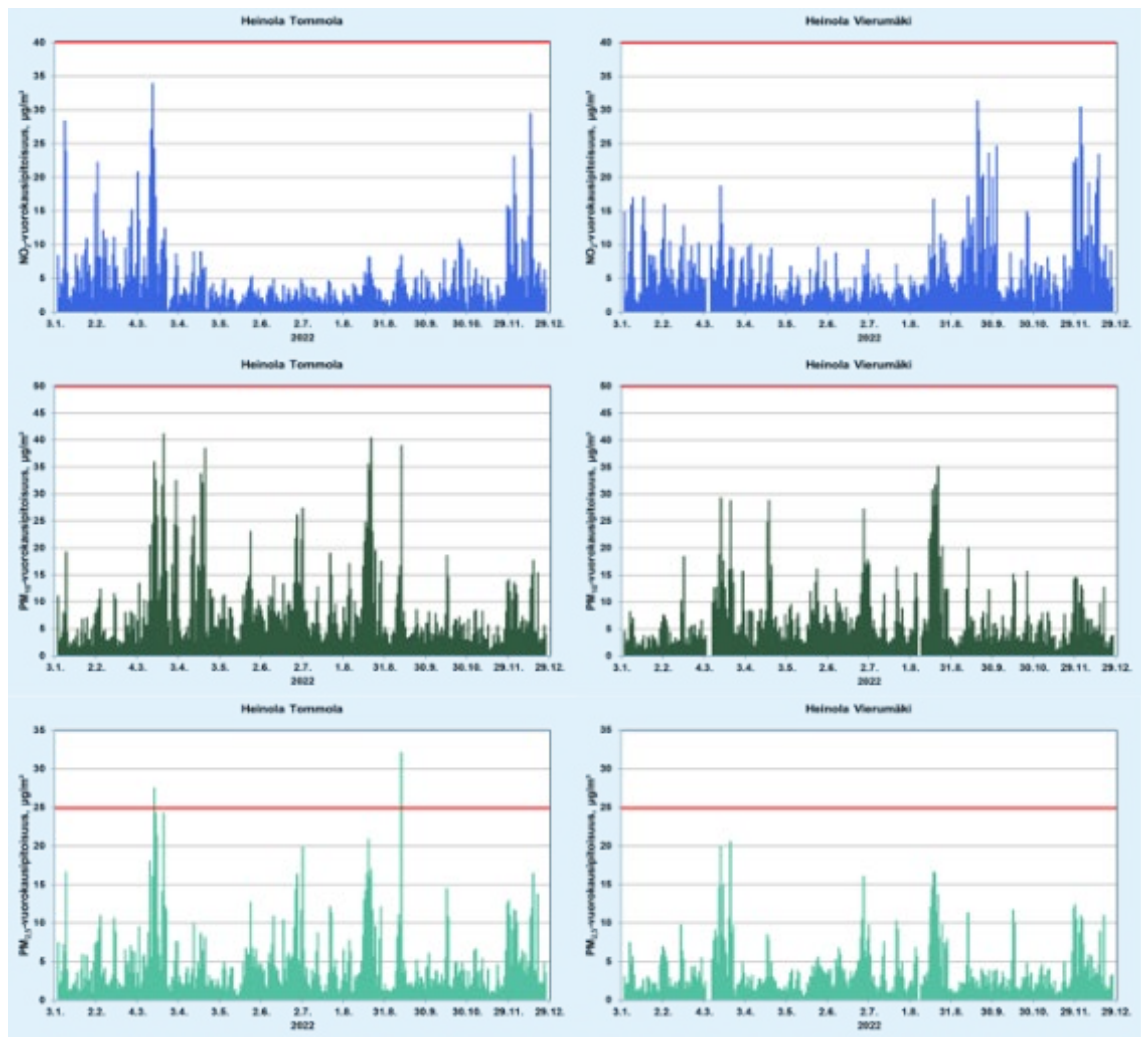
Kuva 2. Heinolan ilmanlaadun mittauspisteissä vuonna 2022 mitatut typpidioksidin (NO 2 ), hengitettävien hiukkasten (PM 10 ) ja pienhiukkasten (PM 2,5 ) vuorokausipitoisuudet. Kuvaajiin on punaisilla vaakaviivoilla merkitty ilmanlaadun raja-arvotasoja.
