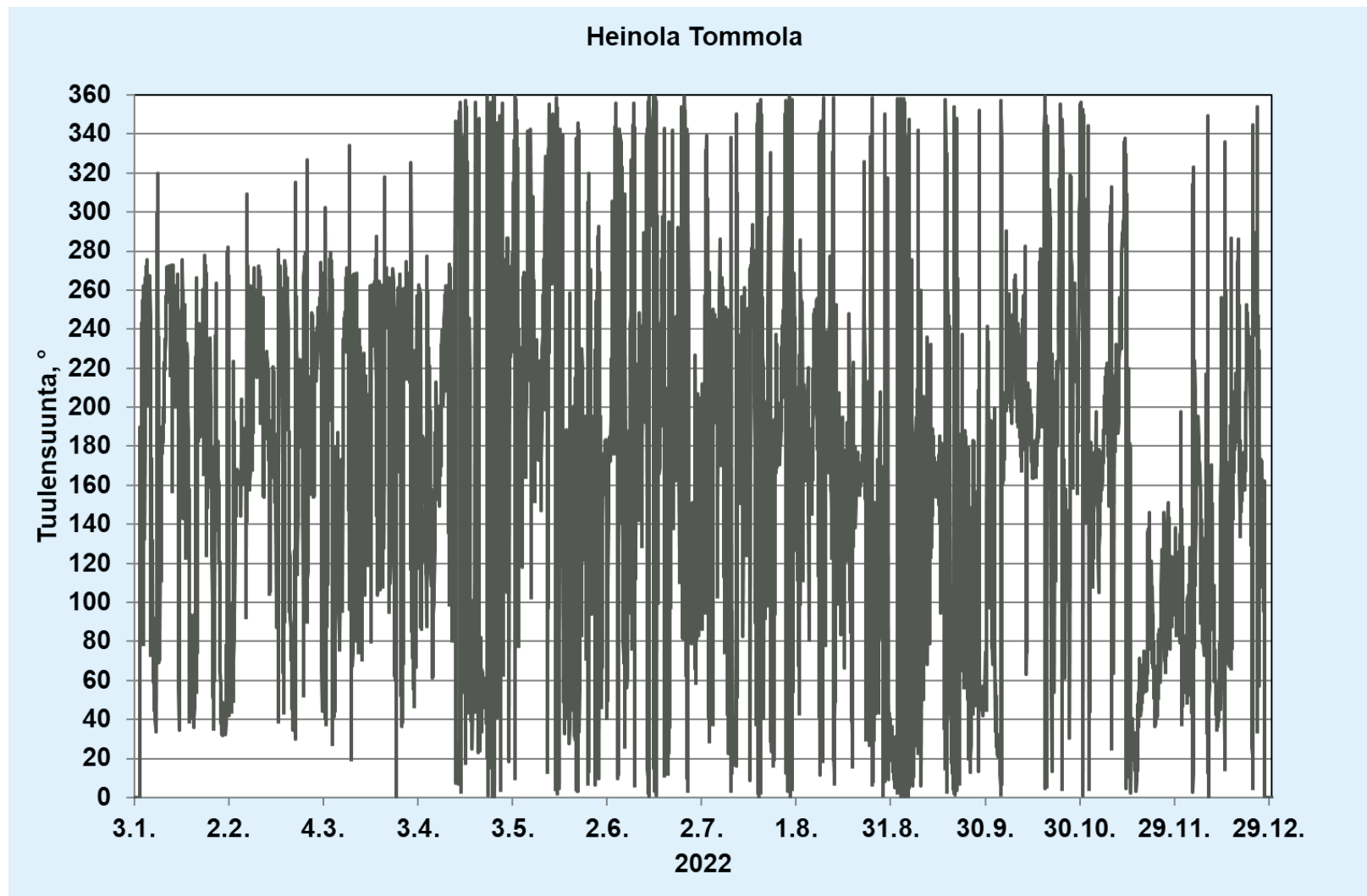
Liitekuva 21. Tuulen suunta (asteina 0–360 °) Heinolan Tommolan mittauspisteessä vuonna 2022.
