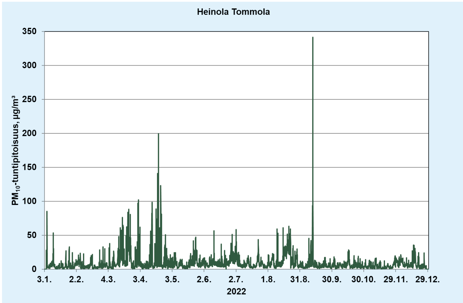
Liitekuva 7. Hengitettävien hiukkasten (PM 10 ) tuntipitoisuudet Heinolan Tammolan mittauspisteessä vuonna 2022.
