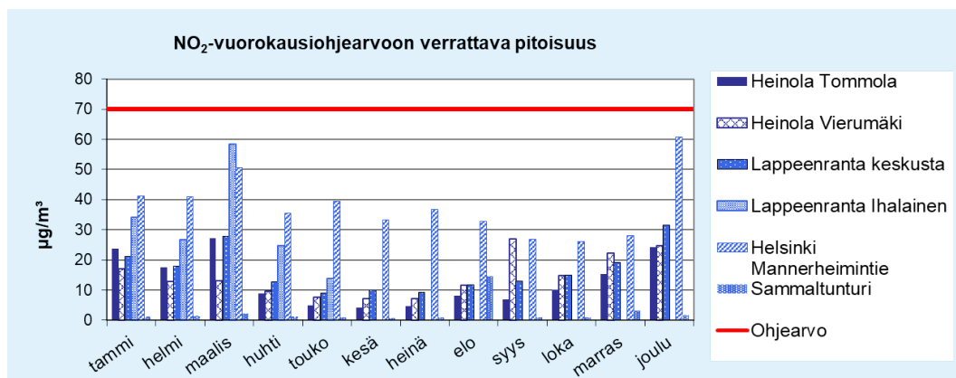
Kuva 19. Typpidioksidipitoisuuden vuorokausiohjeeseen verrattavat pitoisuudet ( \mu\text{g}/\text{m}^3 ) kuukausittain vuonna 2022 eri mittausasemilla. Vuorokausiohjearvo 70 \mu\text{g}/\text{m}^3 on esitetty punaisella vaakaviivalla. Muiden mittausasemien kuin Heinolan pitoisuustulokset ovat vielä tarkistamattomia aineistoa.
