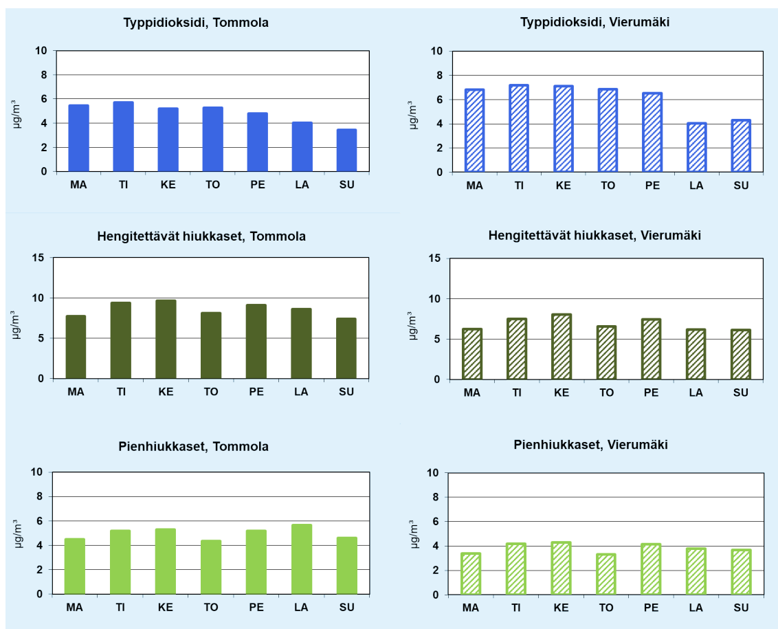
Kuva 14. Heinolan ilmanlaadun mittausasemilla vuonna 2022 mitattujen pitoisuuksien keskiarvot viikonpäivän mukaan.
