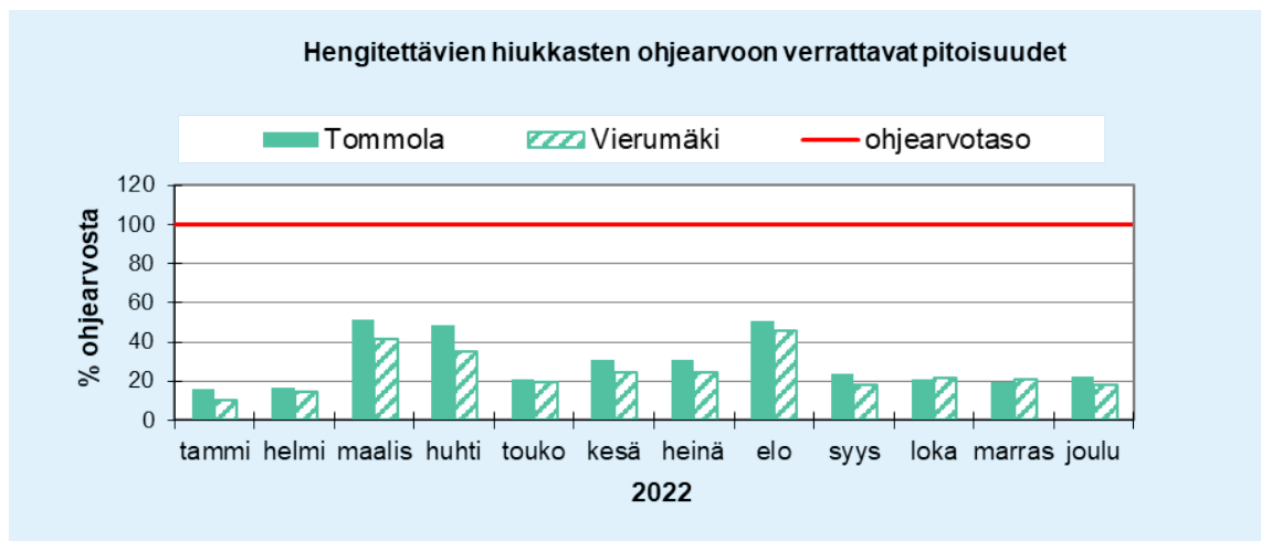
Kuva 9. Hengitettävien hiukkasten ohjearvoon verrattavat pitoisuudet kuukausittain Heinolan ilmanlaadun mittausasemilla vuonna 2022. Punaisella vaakaviivalla (100 %) on merkitty ohjearvotaso 70 \mu\text{g}/\text{m}^3 .
