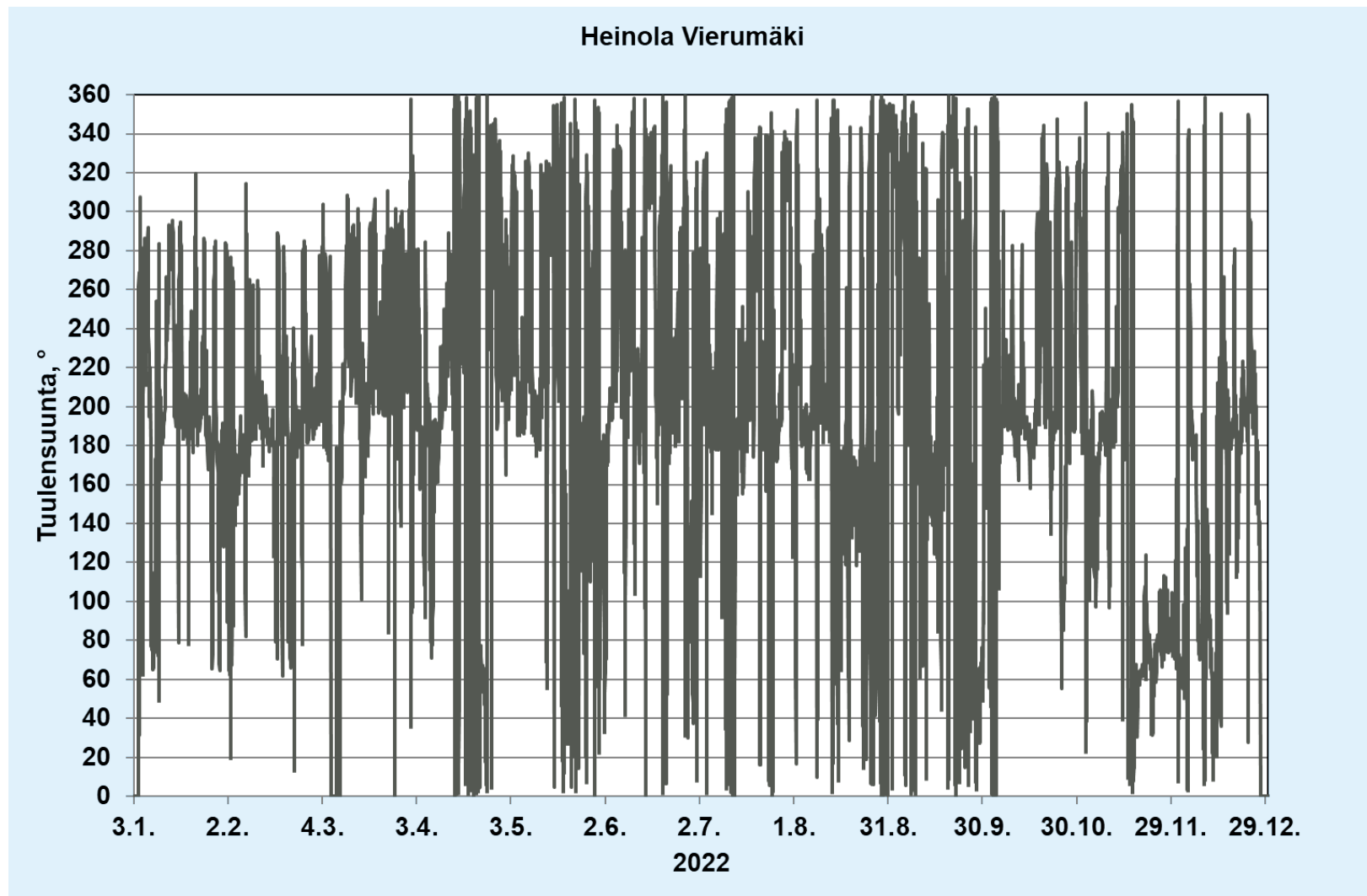
Liitekuva 22. Tuulen suunta (asteina 0–360 °) Heinolan Vierumäen mittauspisteessä vuonna 2022.
