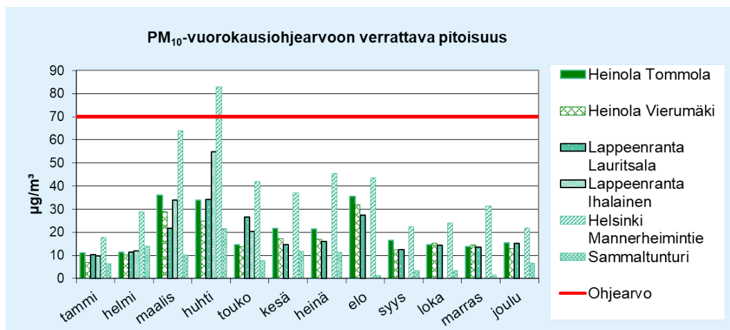
Kuva 20. Hengitettävien hiukkasten pitoisuuden vuorokausiohjeeseen verrattavat pitoisuudet ( \mu\text{g}/\text{m}^3 ) kuukausittain vuonna 2022 eri mittausasemilla. Vuorokausiohjearvo 70 \mu\text{g}/\text{m}^3 on esitetty punaisella vaakaviivalla. Muiden mittausasemien kuin Heinolan pitoisuustulokset ovat vielä tarkistamattomia aineistoa. Lappeenranta Ihalaisen aineisto puuttui ajalta kesä-joulukuu.
