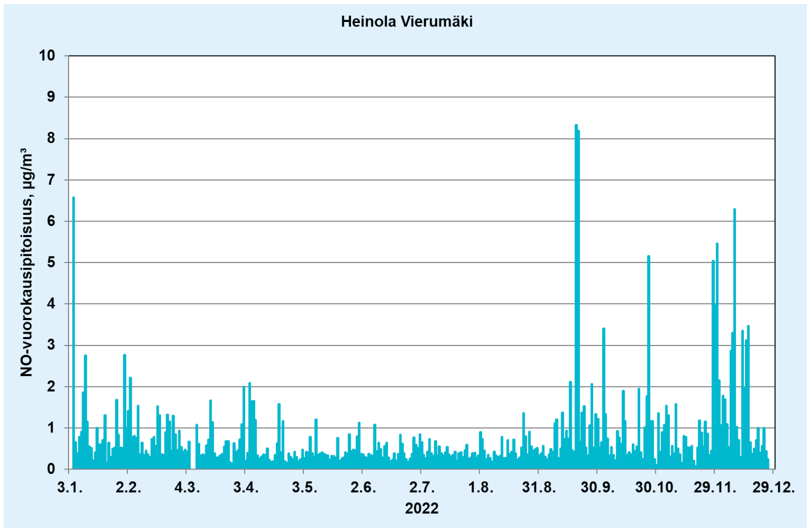
Liitekuva 12. Typpimonoksidin (NO) vuorokausipitoisuudet Heinolan Vierumäen mittauspisteessä vuonna 2022.
