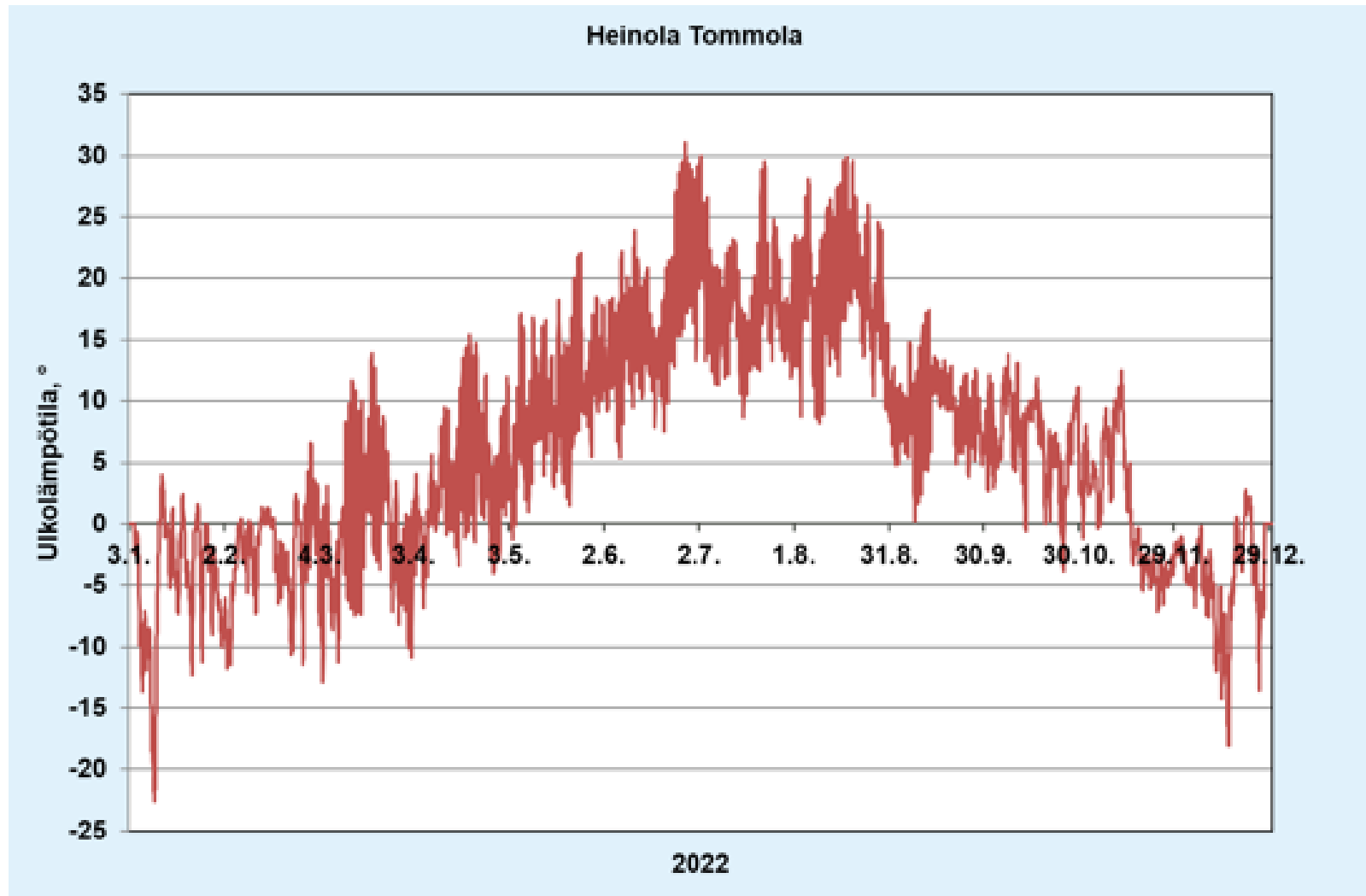
Liitekuva 25. Ulkolämpötila (C °) Heinolan Tommolan mittauspisteessä vuonna 2022.
