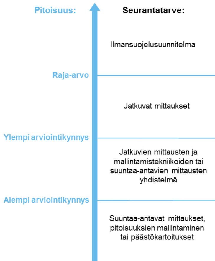
Kuva 38. Ilmanlaadun seurantatarve seuranta-alueella määräytyy mitattujen pitoisuuksien suhteesta ylempään ja alempaan arviointikynnykseen. Seurantatarve kasvaa pitoisuuksien kasvaessa.
