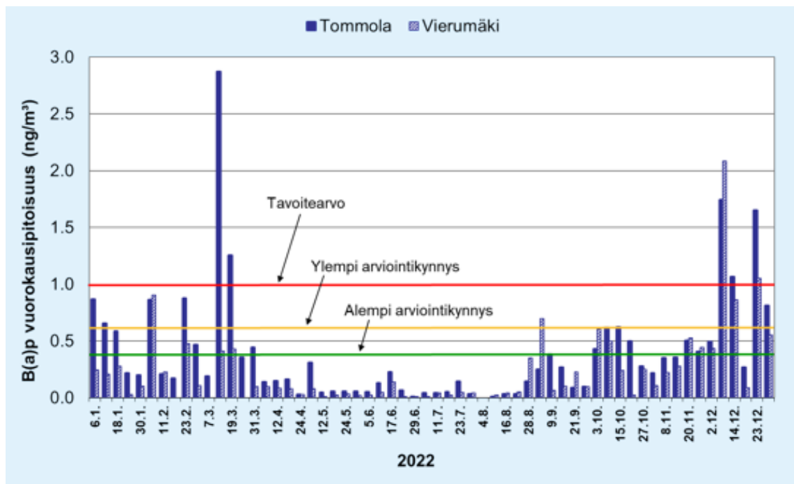
Kuva 15. Hengitettävistä hiukkasista (PM 10 ) määritetyt bentso(a)pyreenin pitoisuudet (ng/m 3 ) Tommolan ja Vierumäen mittauspisteissä vuonna 2022. Kuvaan merkityt tavoitearvo ja arviointikynnykset koskevat vuosikeskiarvoa, eivät yksittäisiä pitoisuusarvoja, ja ne ovat kuvassa vain havainnollistamassa pitoisuustasoa.
