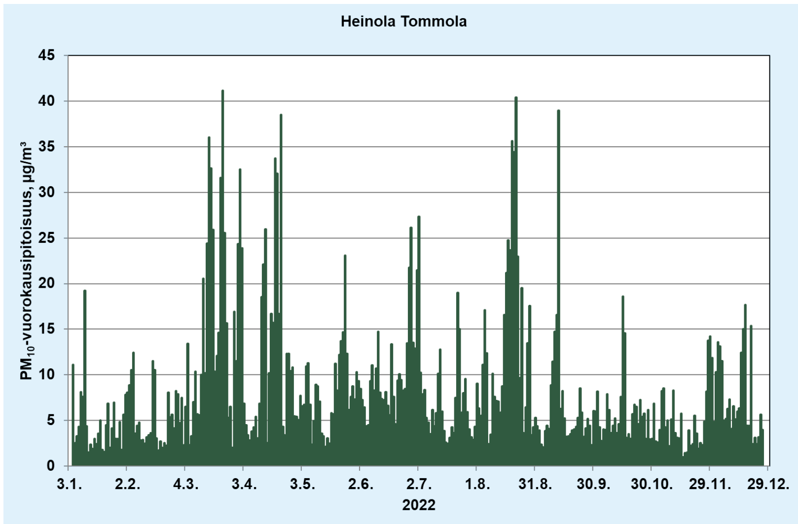
Liitekuva 17. Hengitettävien hiukkasten (PM 10 ) vuorokausipitoisuudet Heinolan Tommolan mittauspisteessä vuonna 2022.
