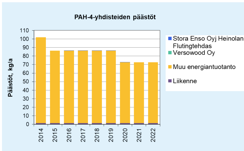
Kuva 36. PAH-4-päästöt Heinolassa vuosina 2014–2022. Stora Enso Oyj:n Heinolan Flutingtehtaan päästöt on esitetty kuvaajassa vuosina 2016–2020 ja Versowood Oy:n vuonna 2016.
