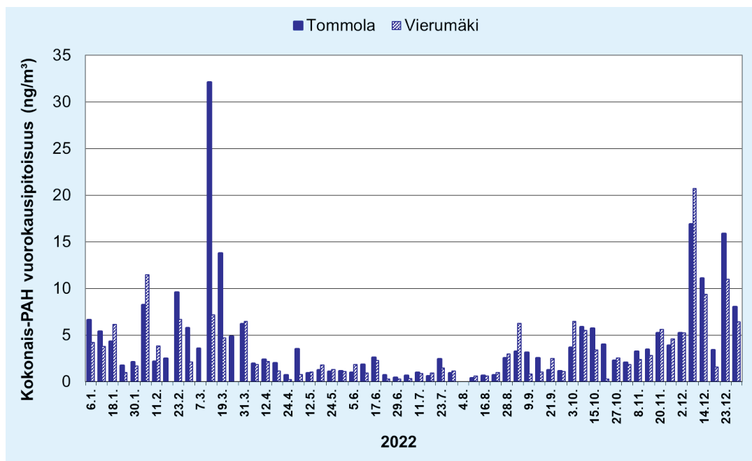
Kuva 16. Hengitettävistä hiukkasista (PM 10 ) määritetyt kokonais-PAH pitoisuudet (ng/m³) Tommolan ja Vierumäen mittauspisteissä vuonna 2022.
