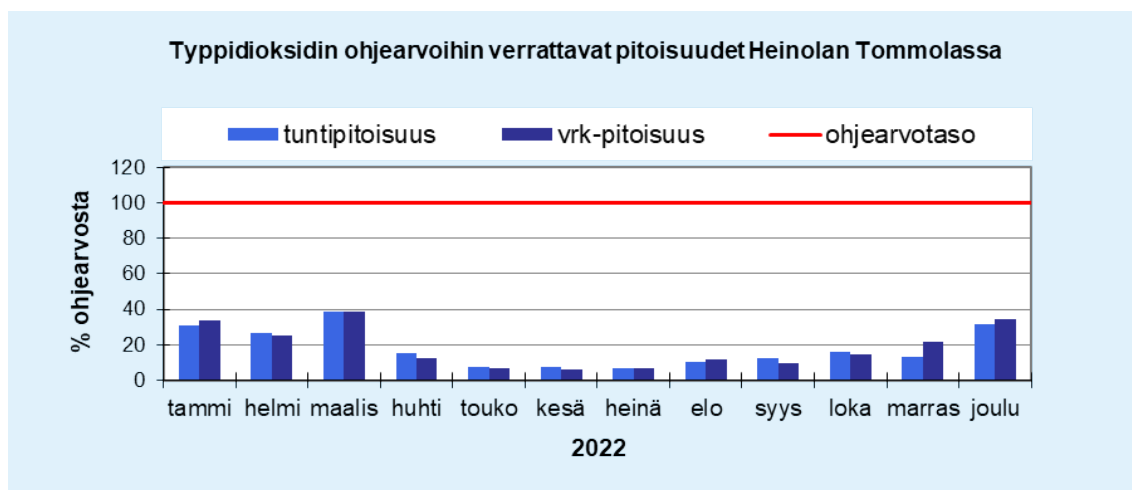
Kuva 7. Typpidioksidin ohjearvoon verrattavat pitoisuudet kuukausittain Heinolan Tommolassa vuonna 2022. Punaisella vaakaviivalla (100 %) on merkitty ohjearvotaso kuukauden tunti- ( 150 \mu\text{g}/\text{m}^3 ) ja vuorokausipitoisuuksille ( 70 \mu\text{g}/\text{m}^3 ).
