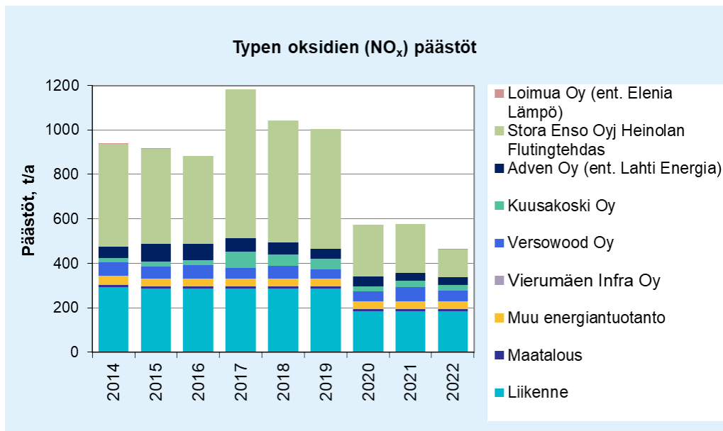
Kuva 34. Typenoksidien päästöt Heinolassa vuosina 2014–2022. Loimua Oy:n päästötiedot on esitetty kuvaajassa vuosina 2014, 2015 ja 2022 ja Vierumäen Infra Oy:n vuodelta 2022 (vuosipäästö 0,05 t/a, joten ei näy kuvaajassa). Tuotteet ja jätteet -päästöluokan päästöosuudet ovat niin pieniä (<0,1 t/a), etteivät ne näy kuvaajassa.
