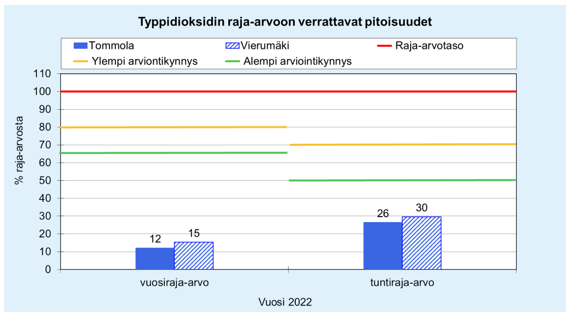
Kuva 4. Typidioksidin raja-arvoon verrattavat pitoisuudet suhteessa (%) raja-arvoihin Heinolan ilmanlaadun mittauspisteissä vuonna 2022. Kuvaan on merkitty vaakaviivoilla raja-arvotaso sekä ylempi ja alempi arviointikynnys.
