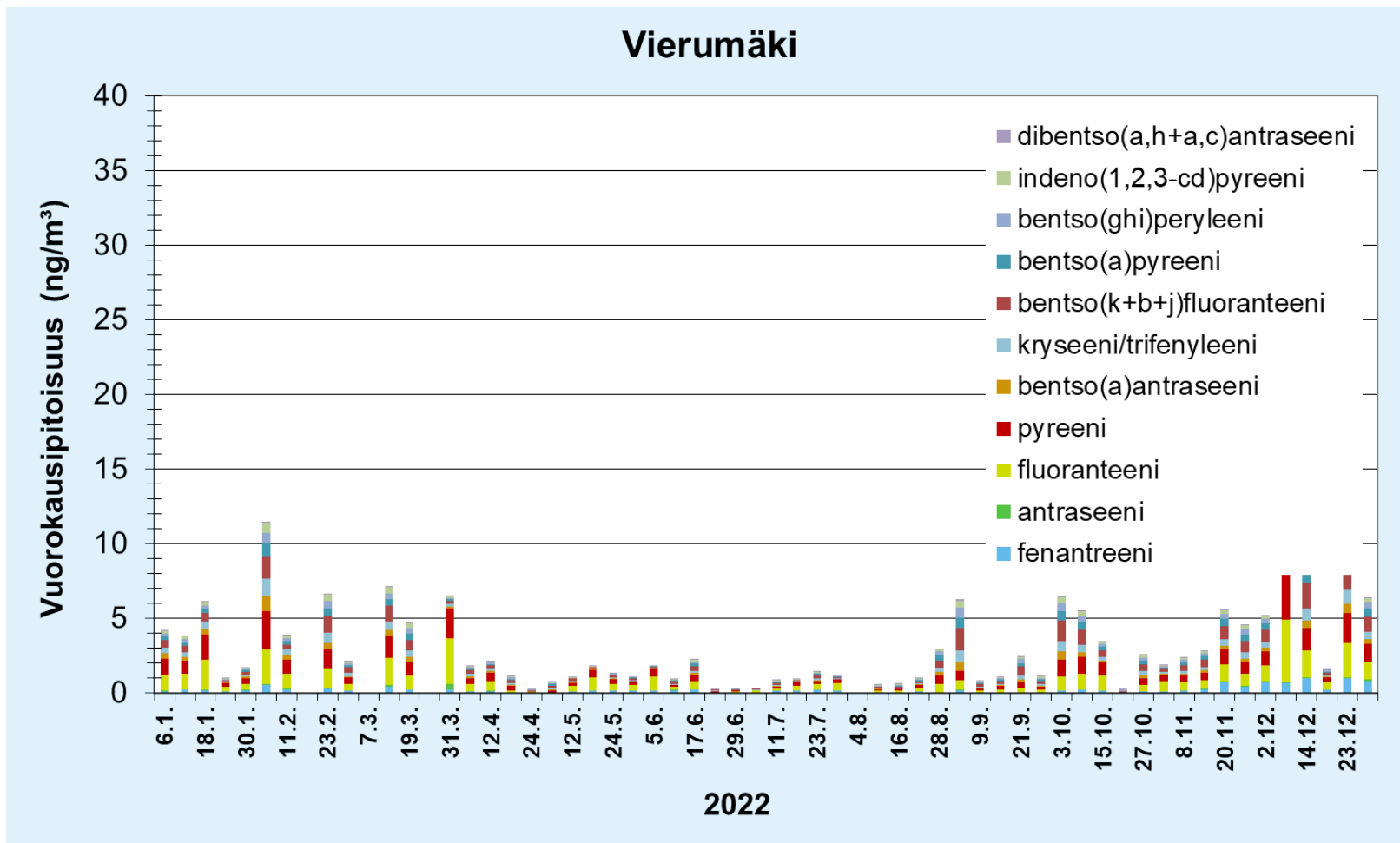
Liitekuva 30. Hengitettävistä hiukkasista (PM 10 ) vuorokausipitoisuudet määritetyt eri PAH-yhdisteiden osuudet kokonaispitoisuuksista (ng/m 3 ) Vierumäen mittauspisteessä vuonna 2022
