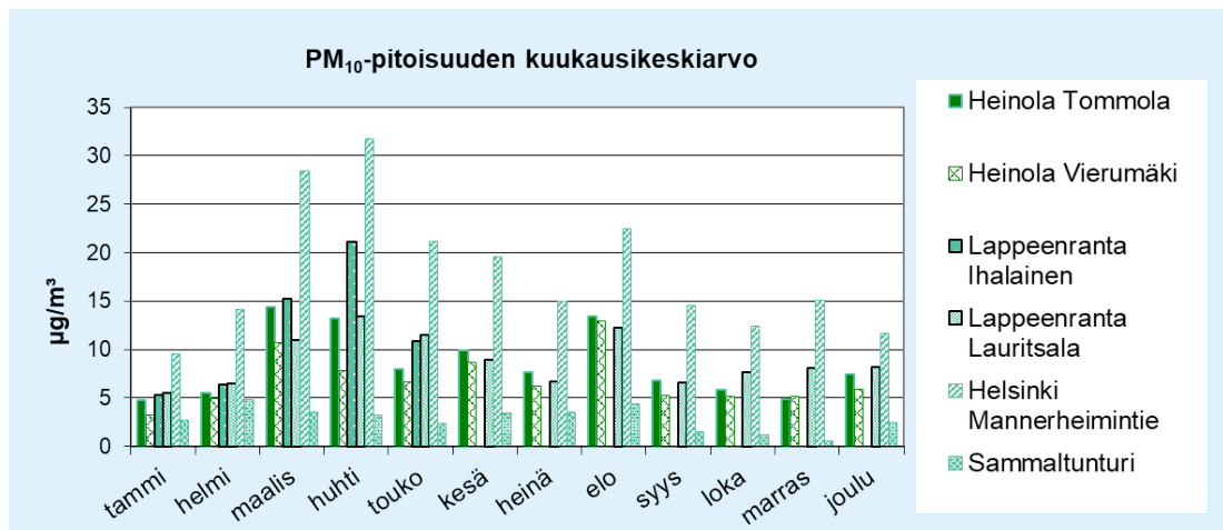
Kuva 22. Heinolan ilmanlaadun mittausasemilla, Lappeenrannan kaupungin mittausasemilla, Helsingin Mannerheimintien mittausasemalla ja Sammalntunturin taustamittausasemalla vuonna 2022 mitatut hengitettävien hiukkasten kuukausikeskiarvopitoisuudet \mu\text{g}/\text{m}^3 .
