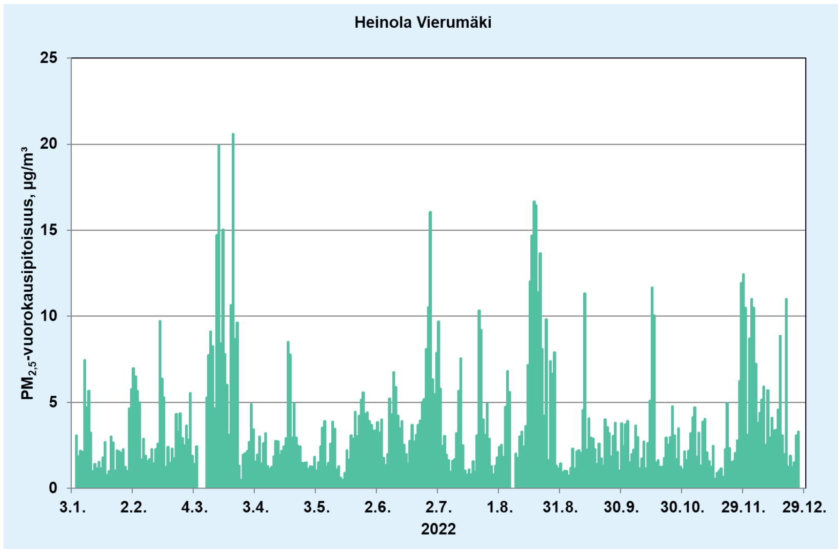
Liitekuva 20. Pienhiukkasten (PM 2,5 ) vuorokausipitoisuudet Heinolan Vierumäen mittauspisteessä vuonna 2022.
