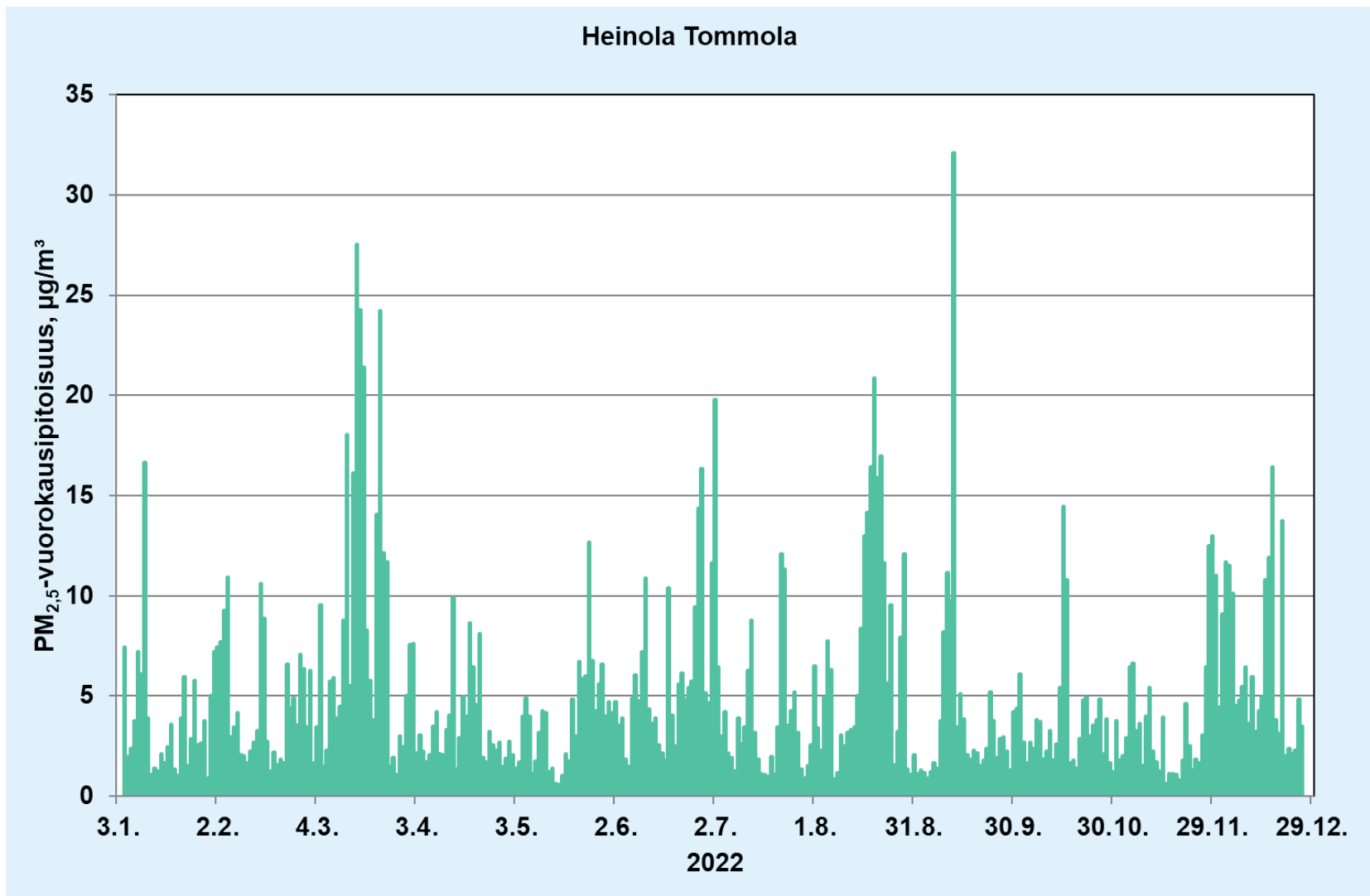
Liitekuva 19. Pienhiukkasten (PM 2,5 ) vuorokausipitoisuudet Heinolan Tommolan mittauspisteessä vuonna 2022.
