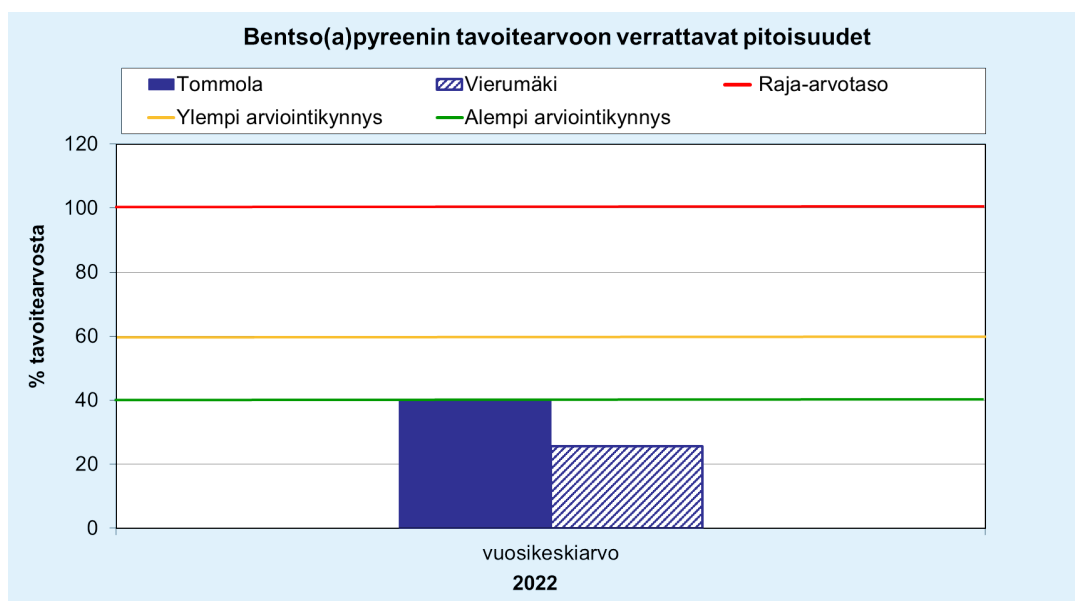
Kuva 17. Bentso(a)pyreenin vuosikeskiarvopitoisuudet suhteessa (%) tavoitearvoon Heinolan Tommolan ja Vierumäen mittauspisteissä vuonna 2022. Kuvaan on merkitty vaakaviivoilla tavoitearvotaso sekä ylempi arviointikynnys ja alempi arviointikynnys.
