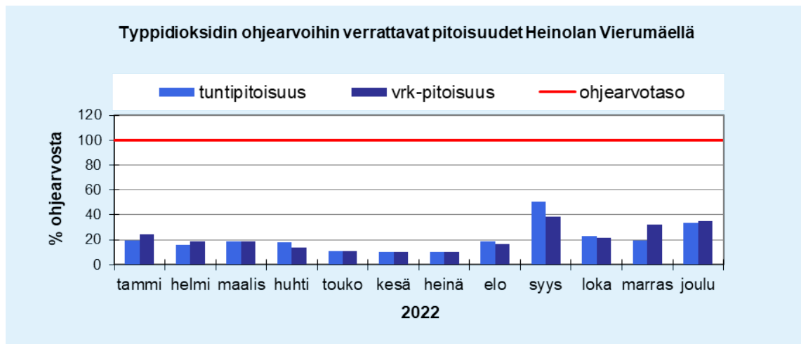
Kuva 8. Typpidioksidin ohjearvoon verrattavat pitoisuudet kuukausittain Heinolan Vierumäellä vuonna 2022. Punaisella vaakaviivalla (100 %) on merkitty ohjearvotaso kuukauden tunti- ( 150 \mu\text{g}/\text{m}^3 ) ja vuorokausipitoisuuksille ( 70 \mu\text{g}/\text{m}^3 ).
