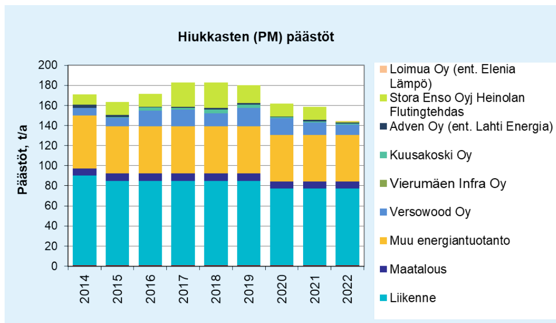
Kuva 35. Hiukkasten päästöt Heinolassa vuosina 2014–2022. Loimua Oy:n (vuosipäästö 0,01 t/a) ja Vierumäen Infra Oy:n (vuosipäästö 0,004 t/a) päästötiedot on esitetty kuvaajassa vain vuonna 2022. Pienet vuosipäästöt eivät näy kuvaajassa.
