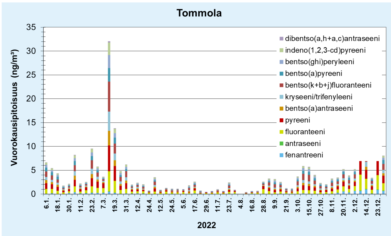
Liitekuva 29. Hengitettävistä hiukkasista (PM 10 ) vuorokausipitoisuudet määritetyt eri PAH-yhdisteiden osuudet kokonaispitoisuuksista (ng/m³) Tommolan mitauspisteessä vuonna 2022.
