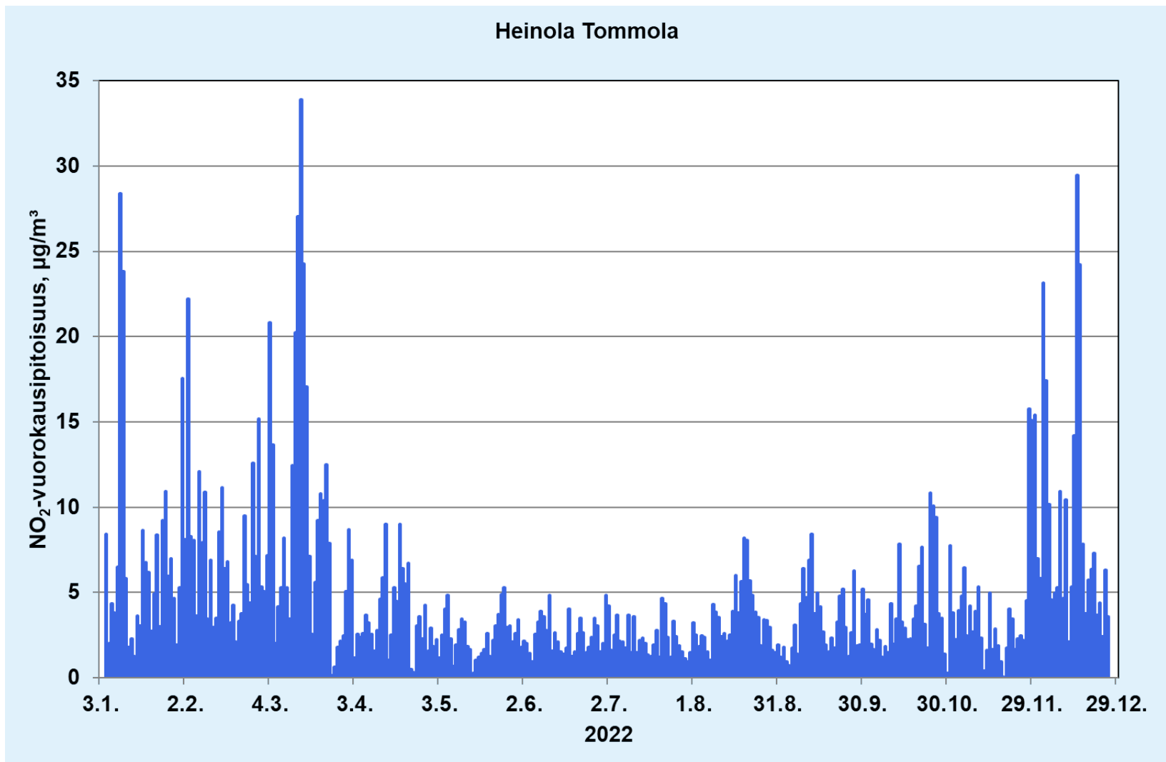
Liitekuva 13. Typpidioksidin (NO 2 ) vuorokausipitoisuudet Heinolan Tommolan mittauspisteessä vuonna 2022.
