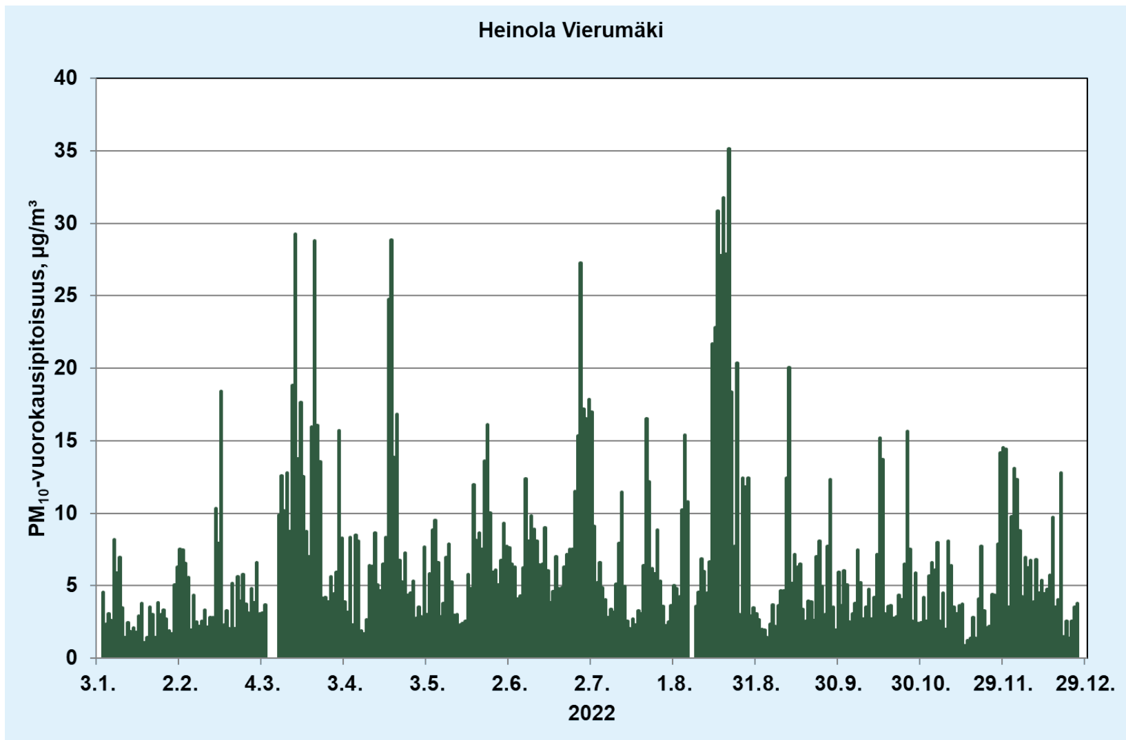
Liitekuva 18. Hengitettävien hiukkasten (PM 10 ) vuorokausipitoisuudet Heinolan Vierumäen mittauspisteessä vuonna 2022.
