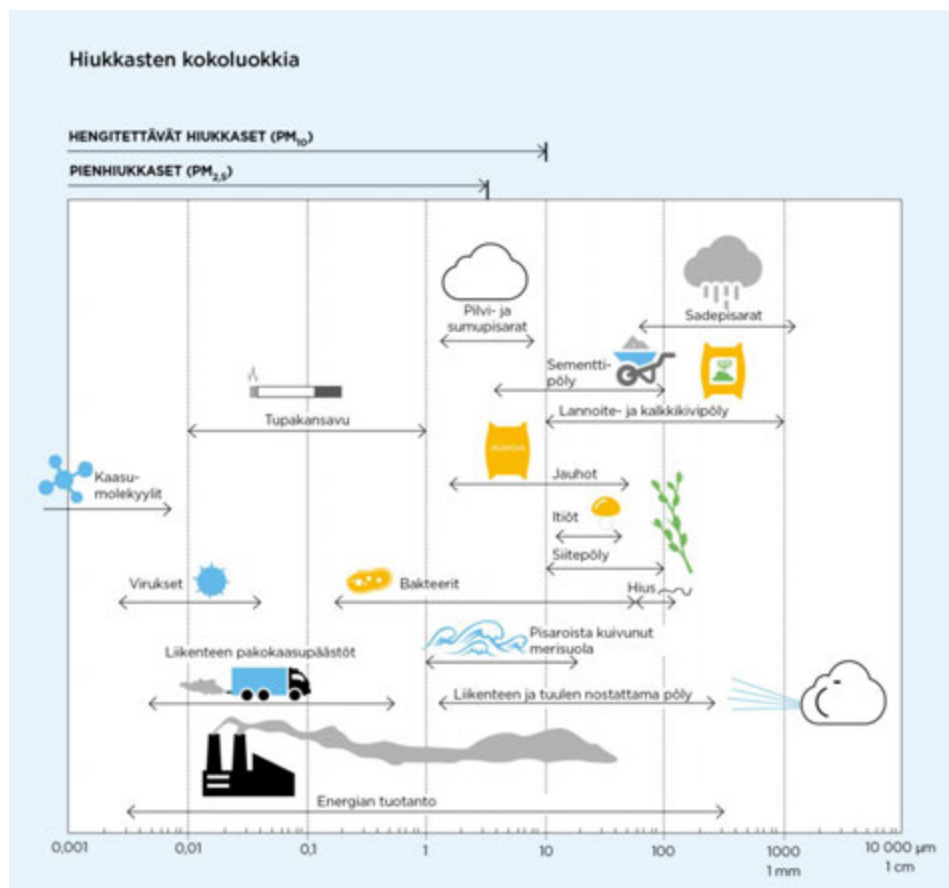
Kuva 47. Hiukkasten kokoluokkia. Hiukkasten koko ilmaistaan halkaisijana mikrometreissä ( \mu\text{m} ). Mikro ( \mu ) etuliite tarkoittaa miljoonasosaa. 1 \mu\text{m} on siten metrin metrin miljoonasosa eli millimetrin tuhannesosa.
