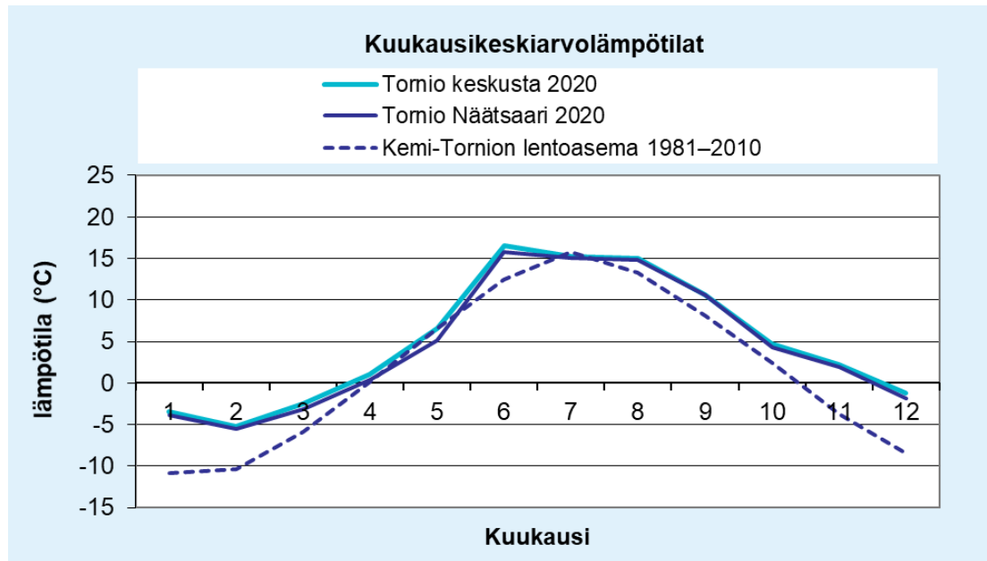
Kuva 38. Lämpötilan kuukausikeskiarvot Tornion keskustassa ja Näätsaassa vuonna 2020, Kemi-Tornion lentoasemalla mitattuihin ilmastollisen vertailukauden 1981–2010 pitkäaikaikeskiarvoihin nähden.
